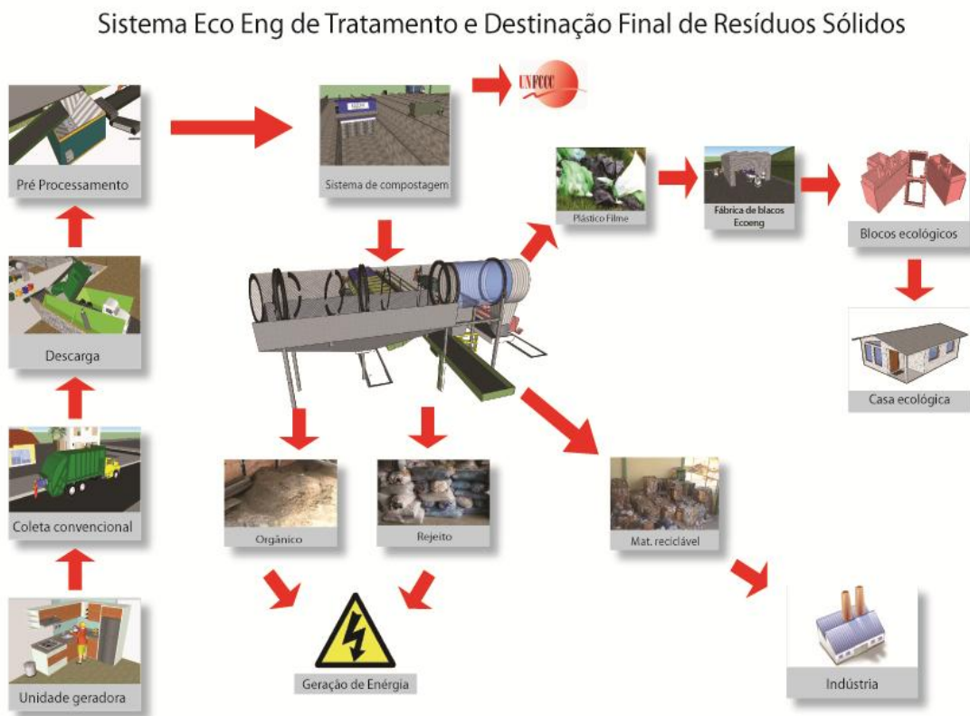
Figura 12: Sistema Eco Eng - Tratamento e destinação Final de Resíduos Sólidos
