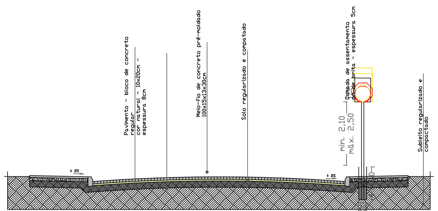
SEÇÃO TIPO - PAVIMENTAÇÃO ESCALA 1:75
