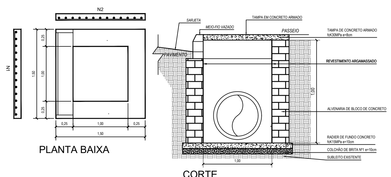
CAIXAS BOCA-DE-LOBO ESCALA 1:25
