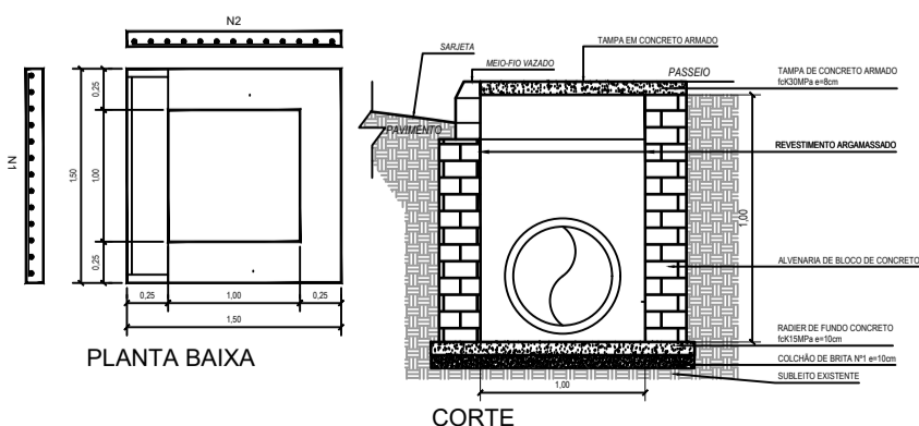
CAIXAS BOCA-DE-LOBO ESCALA 1:25
