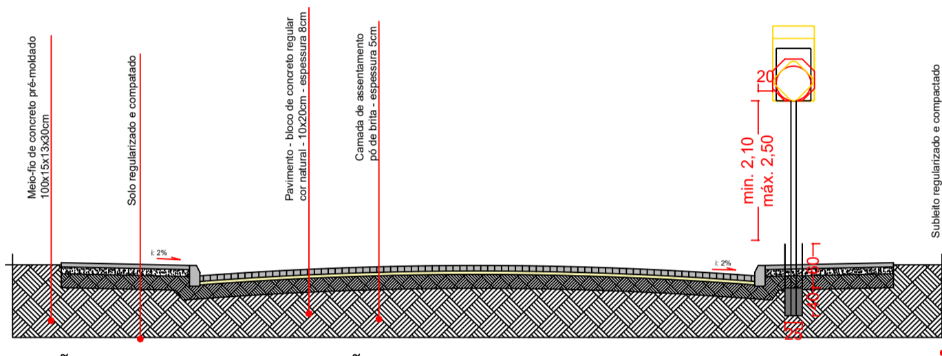
SEÇÃO TIPO - PAVIMENTAÇÃO ESCALA 1:75
