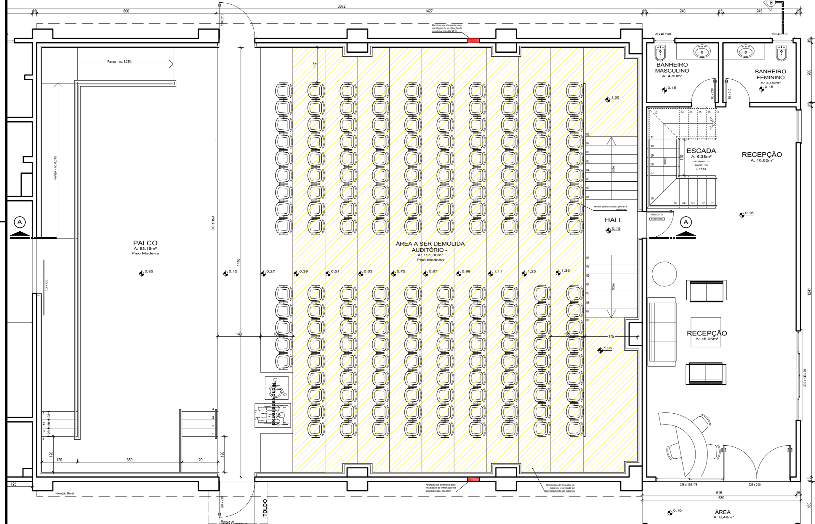
PLANTA BAIXA - INTERVENÇÕES A FAZER TÉRREO A=151,30m² ESCALA: 1/75
