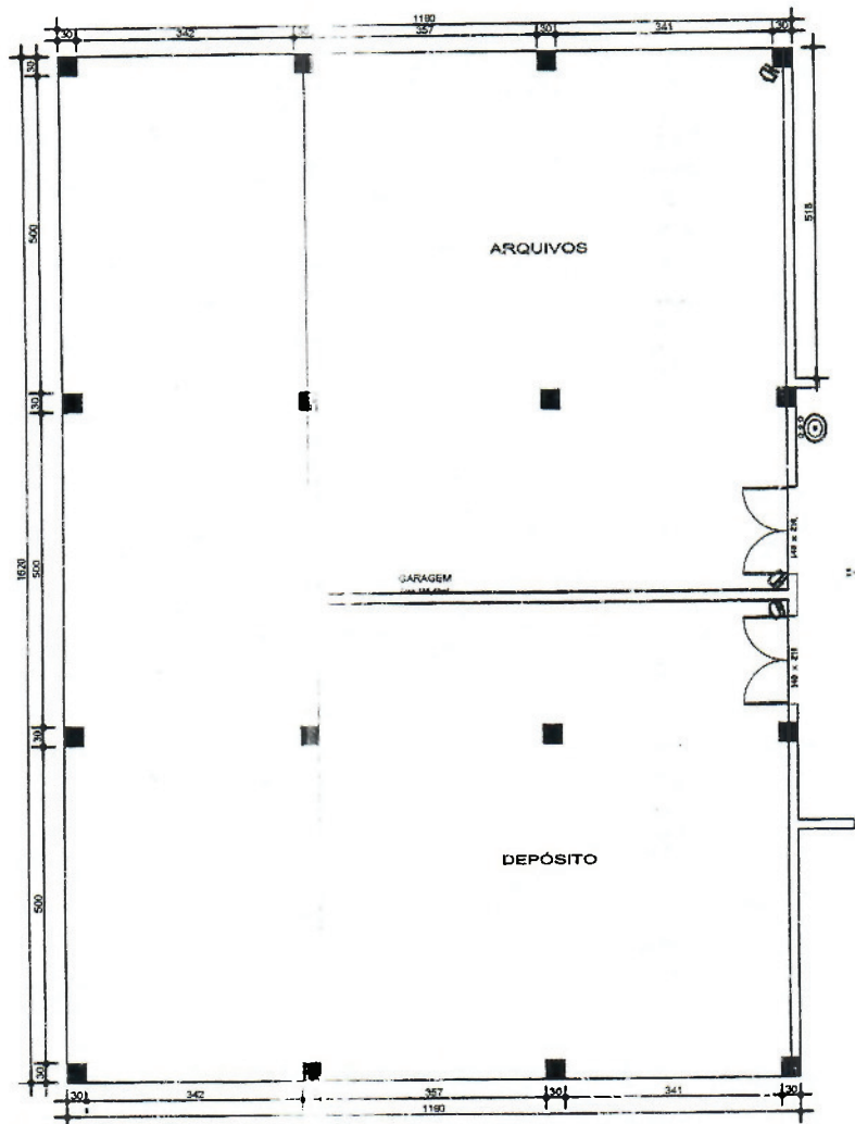
PLANTA BAIXA 2º SUB-SOLO À CONSTRUIR Área: 234,68m 2 esc.: 1/50
