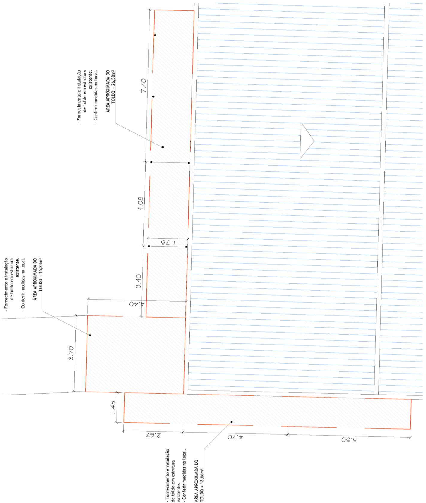
Imagem 01 – Planta Baixa com as medidas do toldo em projeção.
