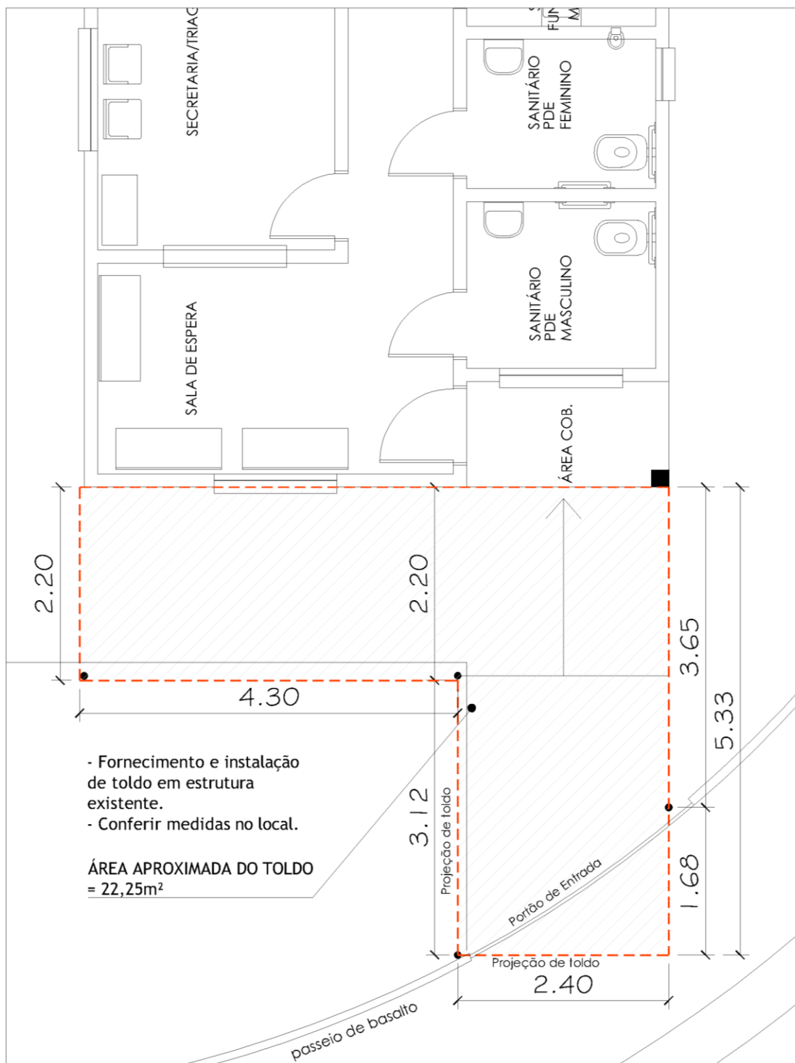
Imagem 01 - Entrada Principal do Posto - Planta Baixa com as medidas do toldo em projeção. OBS.: Conferir todas as medidas no local.
