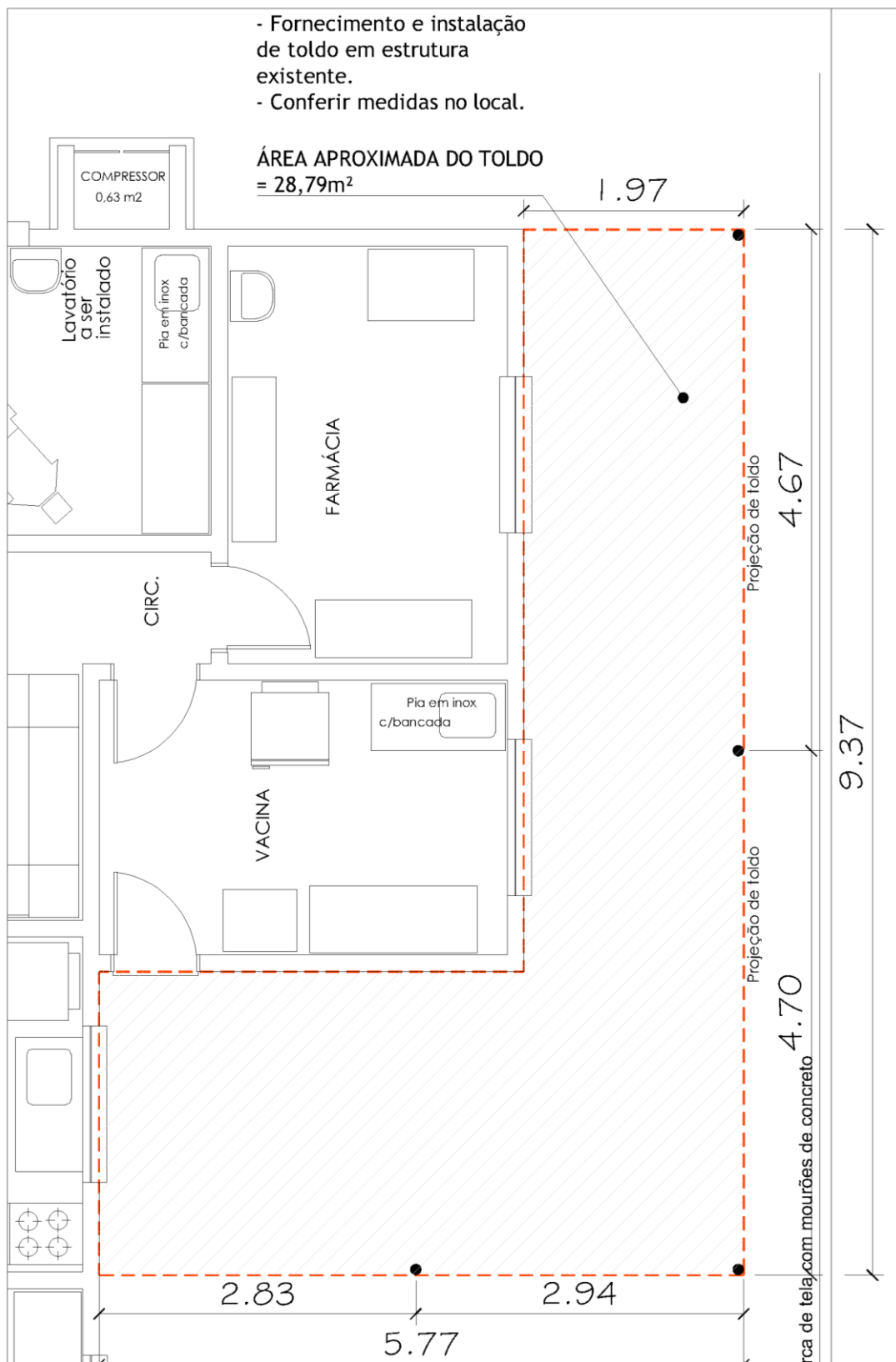
Imagem 02 – Lateral do Posto – Planta Baixa com as medidas do toldo em projeção. OBS.: Conferir todas as medidas no local.
