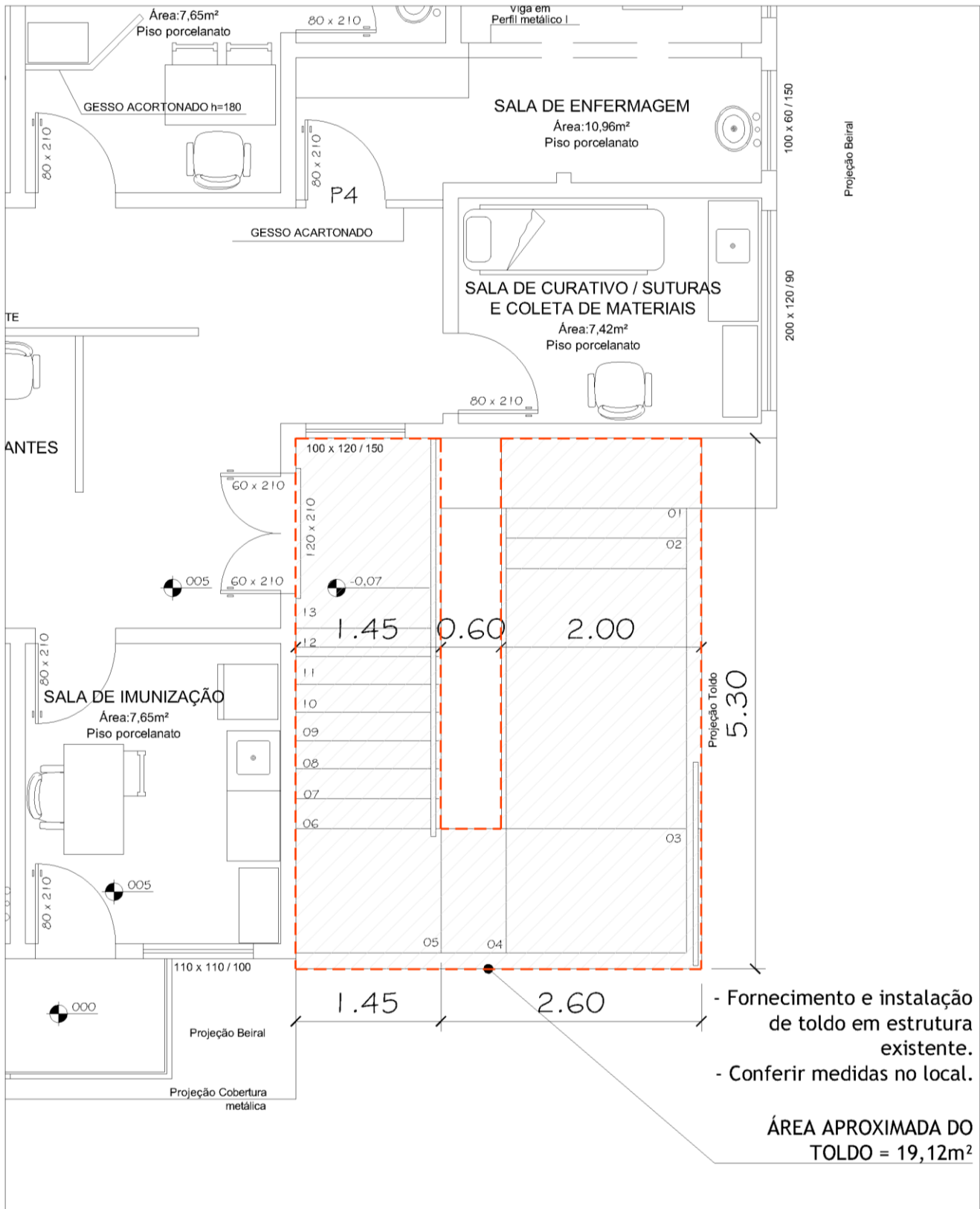
Imagem 01 – Lateral do Posto – Planta Baixa com as medidas do toldo em projeção.
